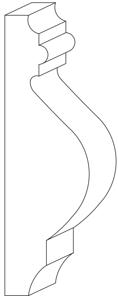
KCW-1516 1-7/16" x 4-11/16"
