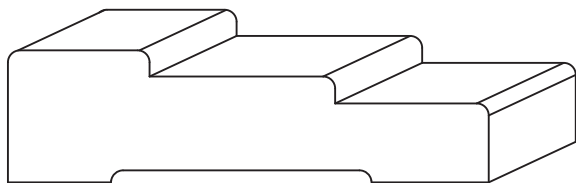
KCW-318 11/16" x 2 1/2"
